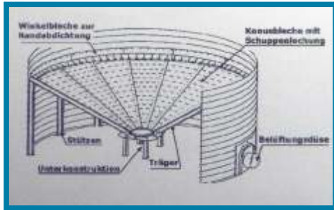
Belüftungskonus
