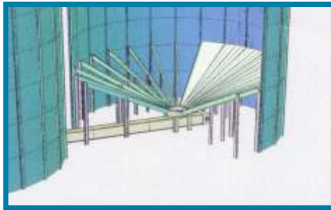
Belüftungskonus im Rundsilo
